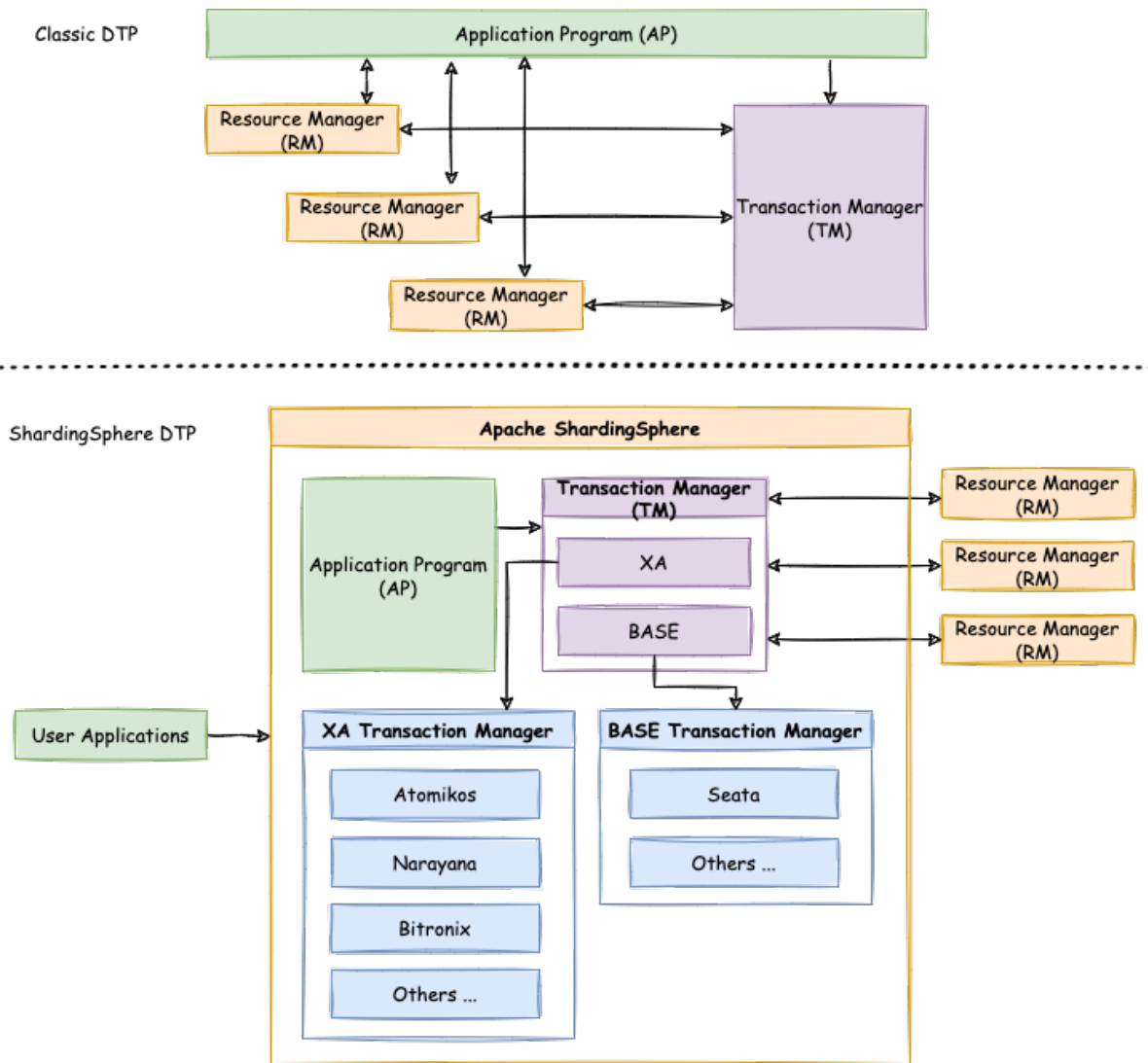
图 4: 两阶段提交模型
