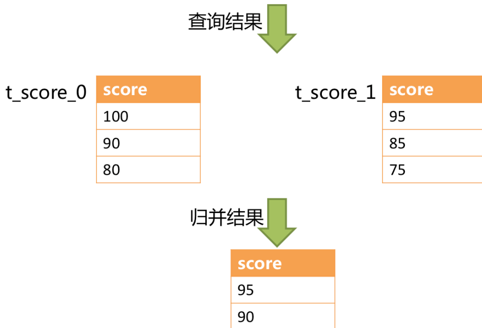
图 5: 改写 SQL 的分页执行结果
