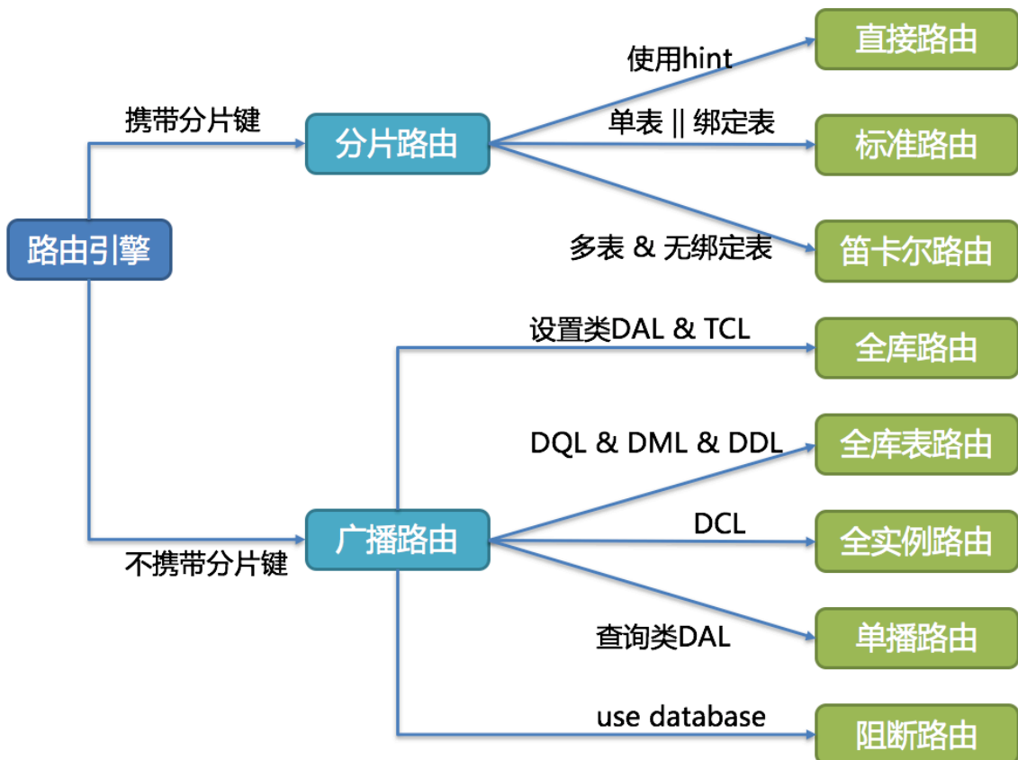
图 3: 路由引擎结构
