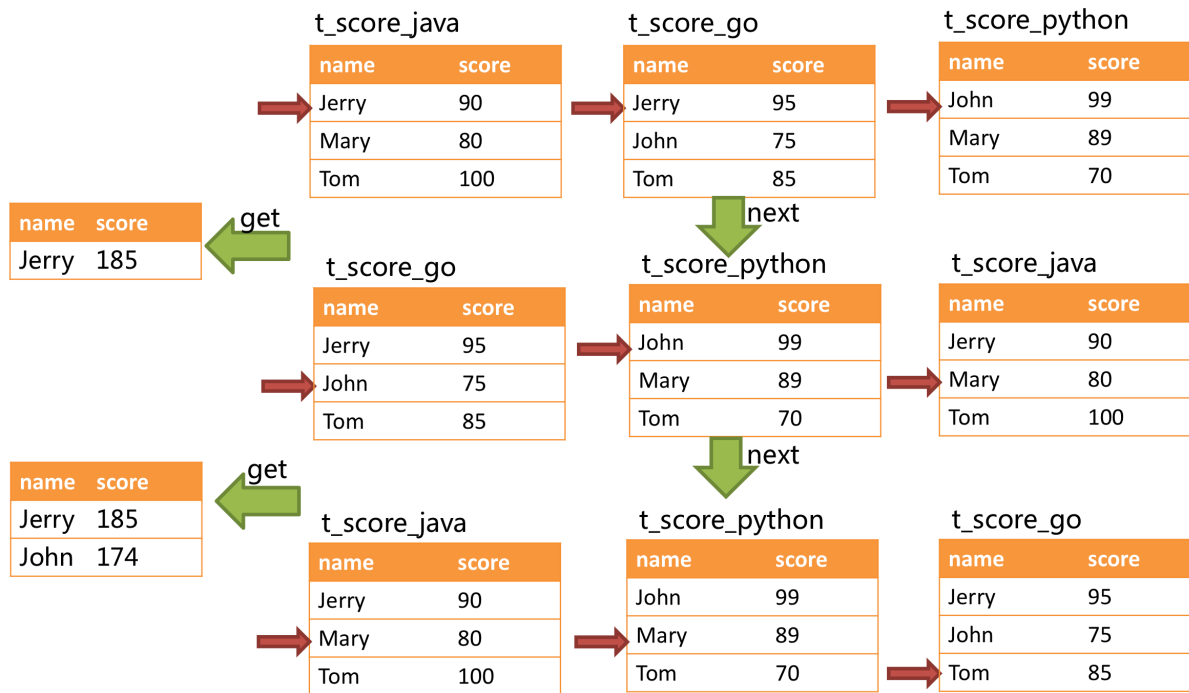
图 13: 分组归并示例 2
