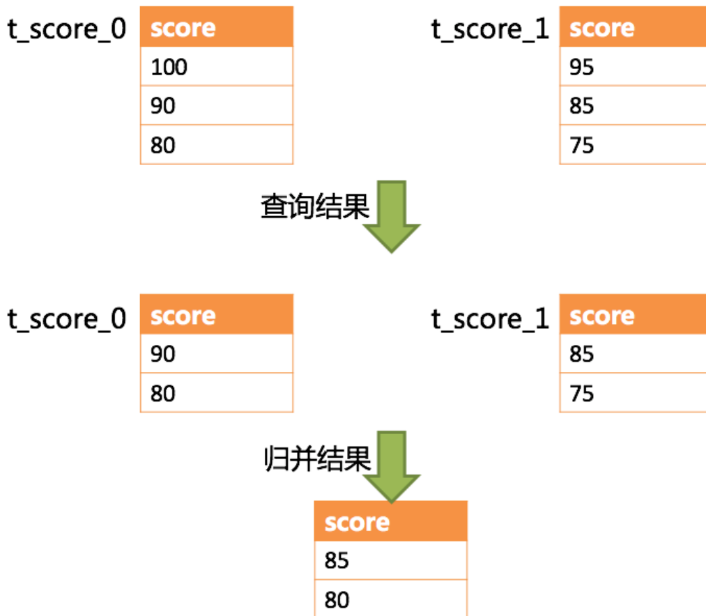
图 4: 不改写 SQL 的分页执行结果
