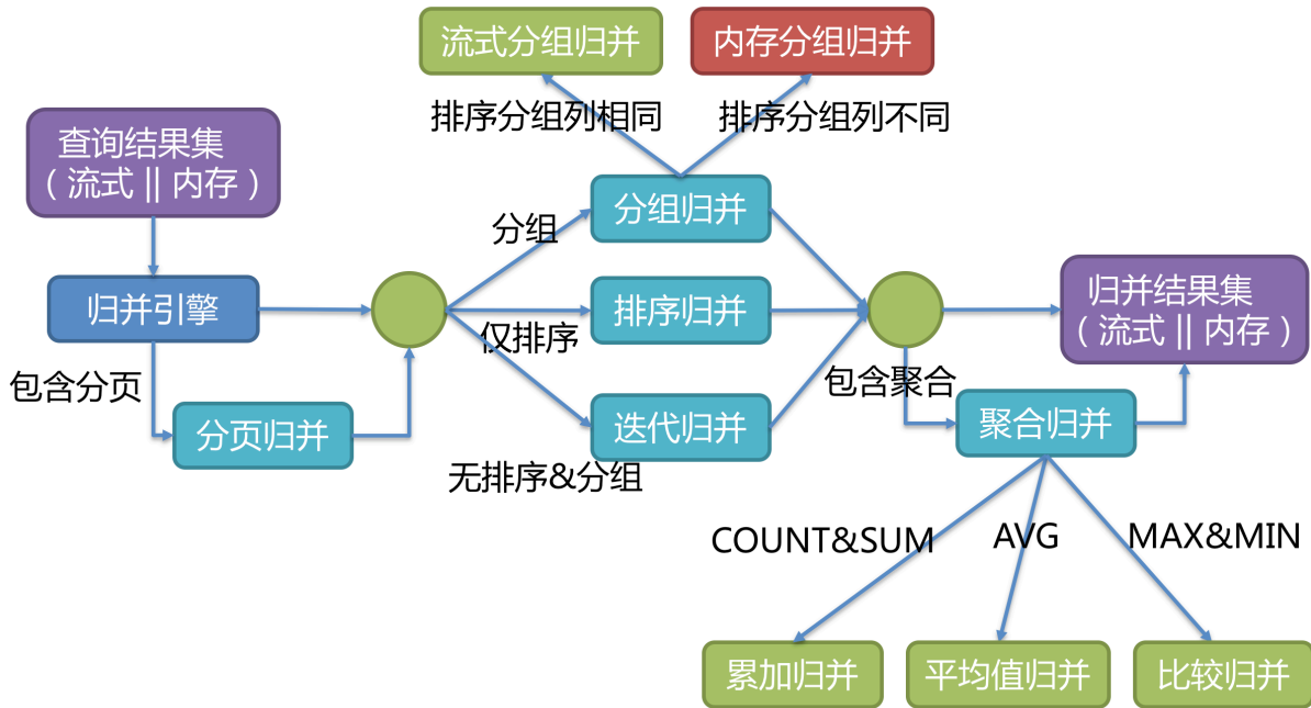
图 14: 归并引擎结构
