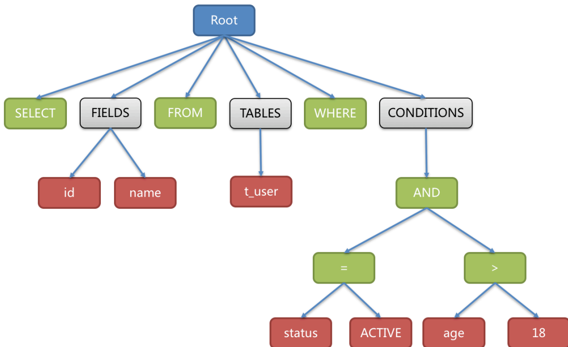
图 2: SQL 抽象语法树
