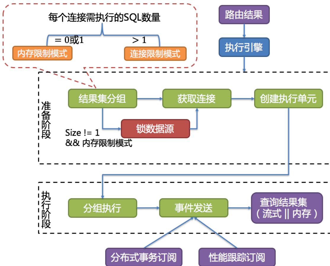
图 9: 执行引擎流程图
