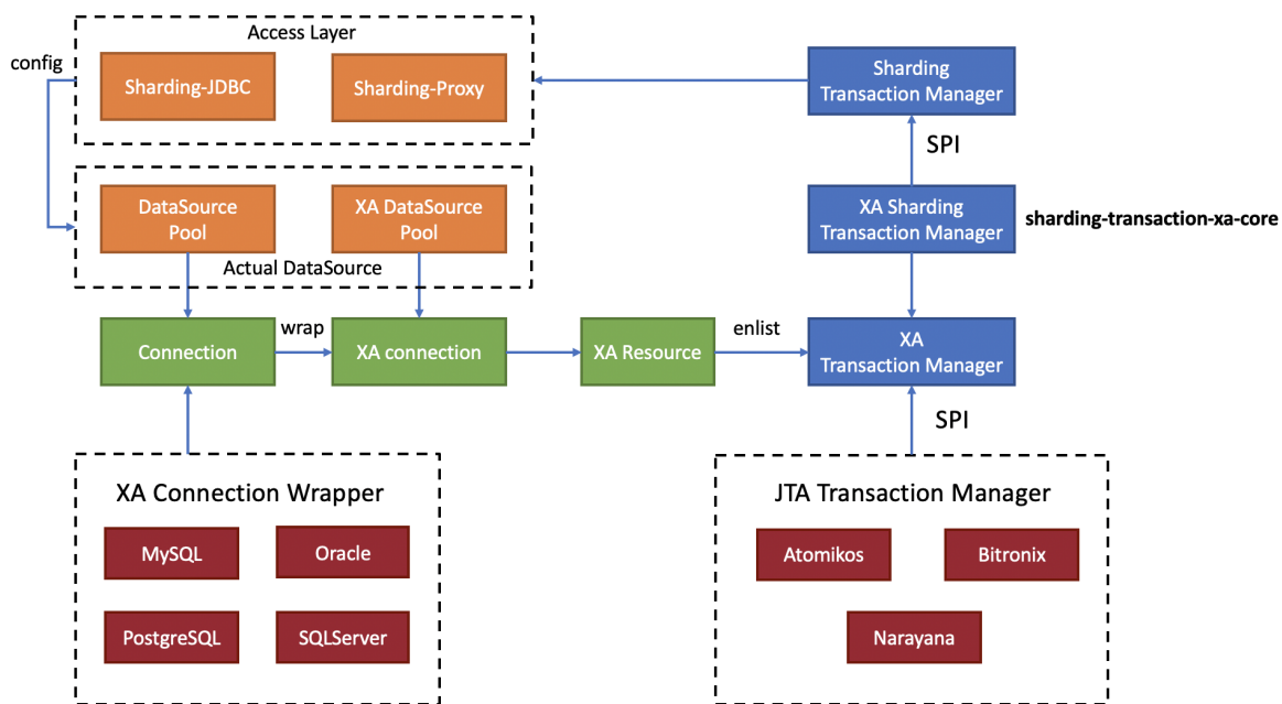
图 15: XA 事务实现原理
