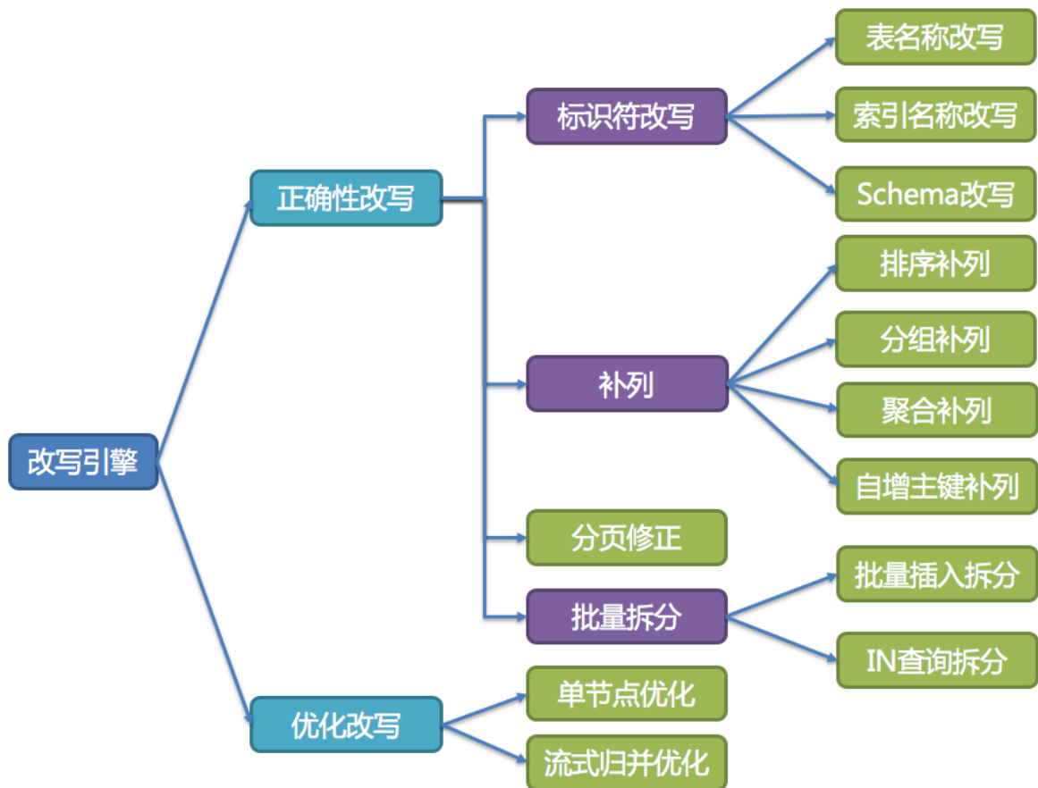
图 6: 改写引擎结构
