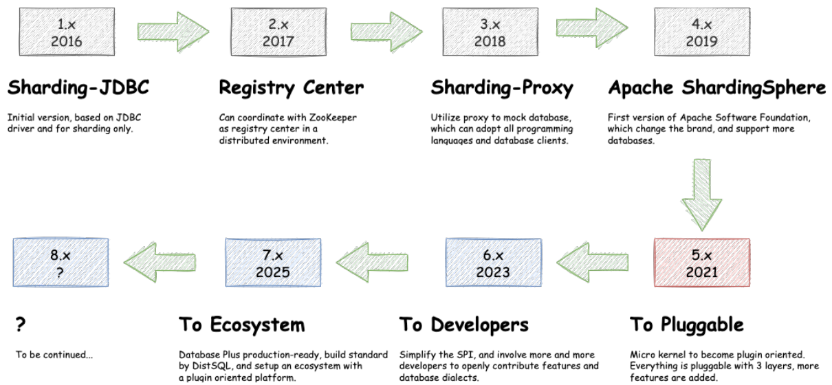
图 1: Roadmap
