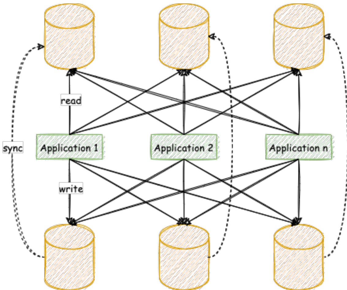
图 6: 挑战
