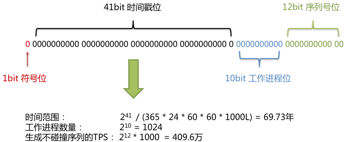
图 3: 雪花算法
