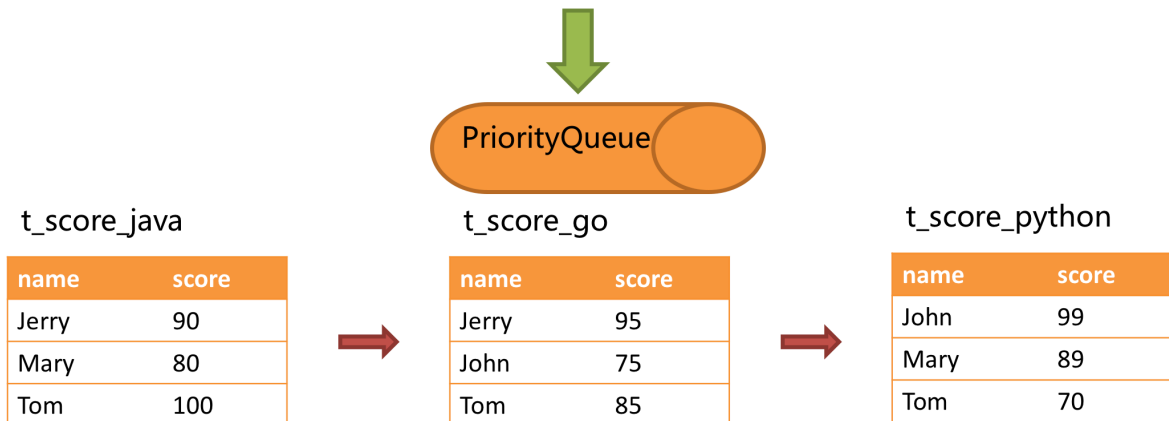
图 12: 分组归并示例 1
